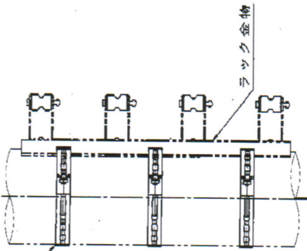
装柱図例
