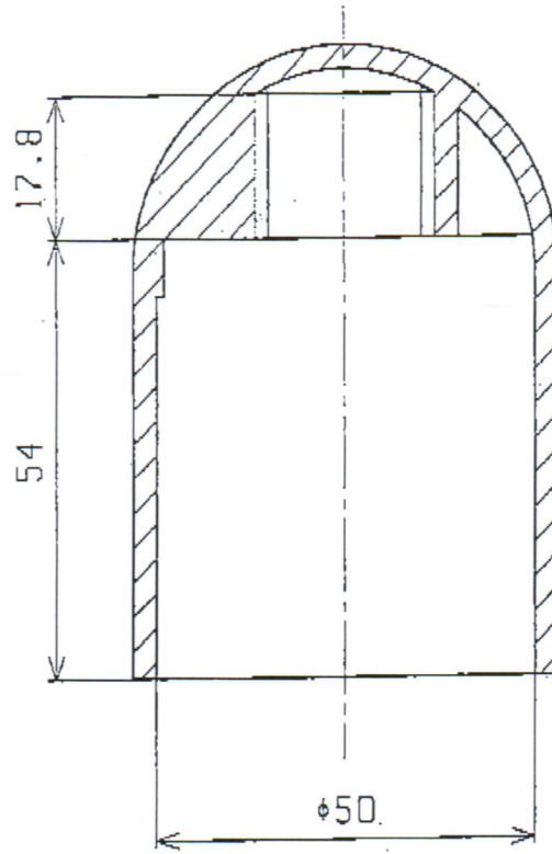
A-A' 断面図
