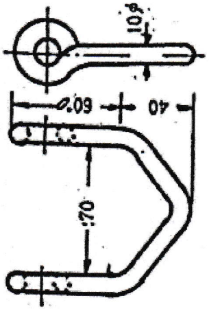
V型ボルト
